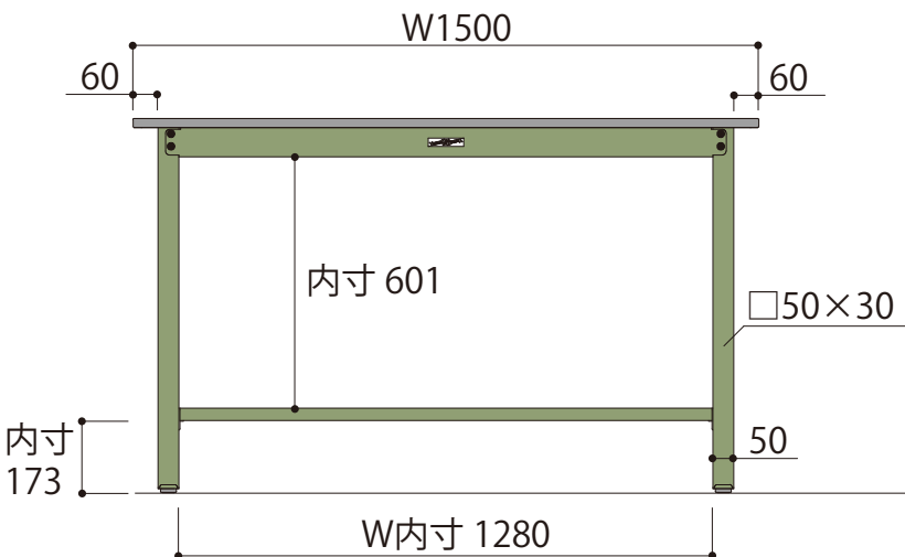
正面図
