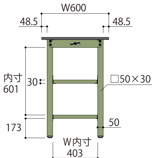
正面図
