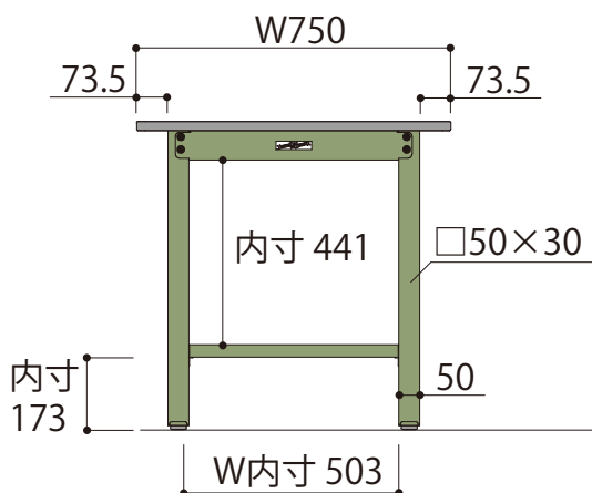
正面図
