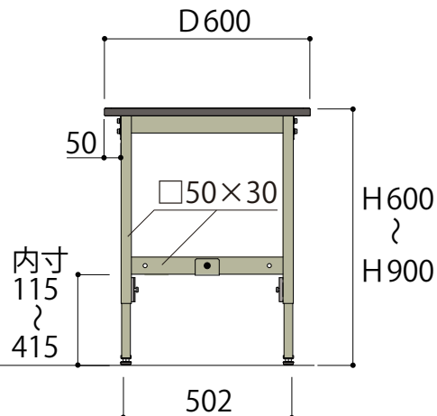
側面図
