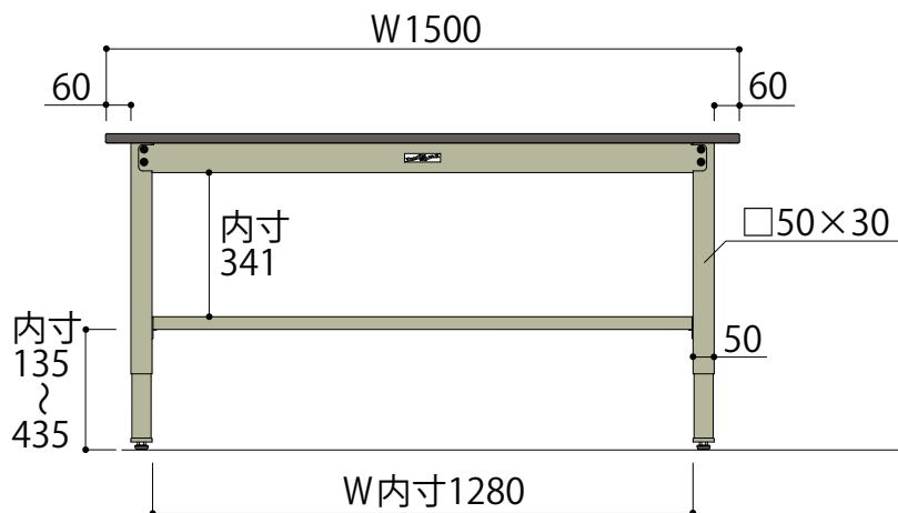
正面図
