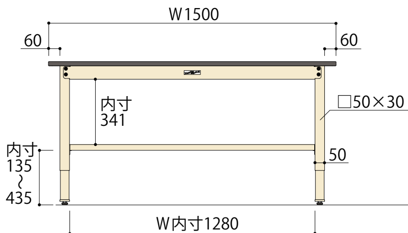
正面図
