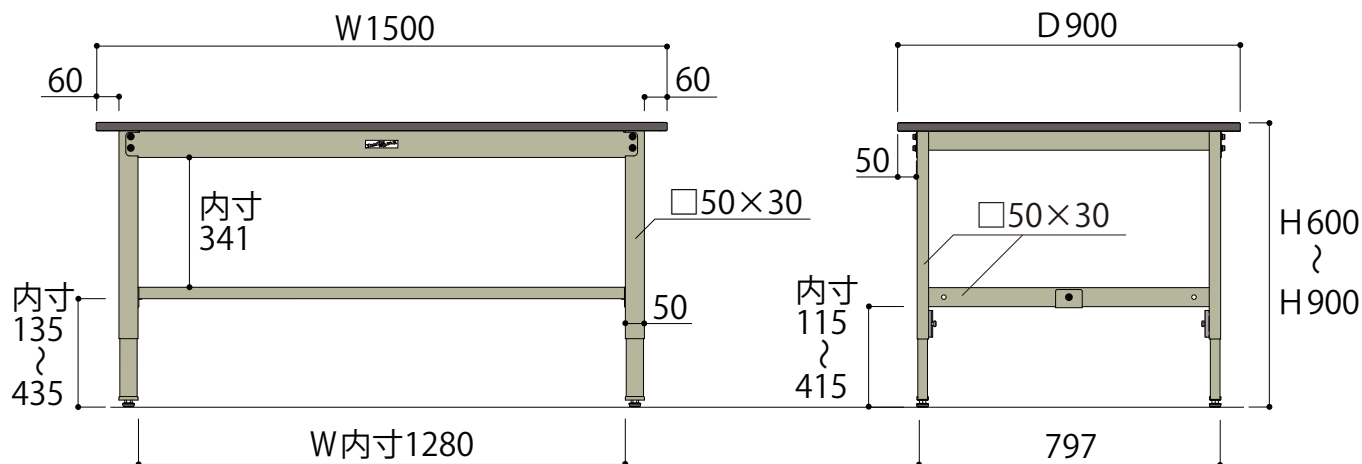
正面図
