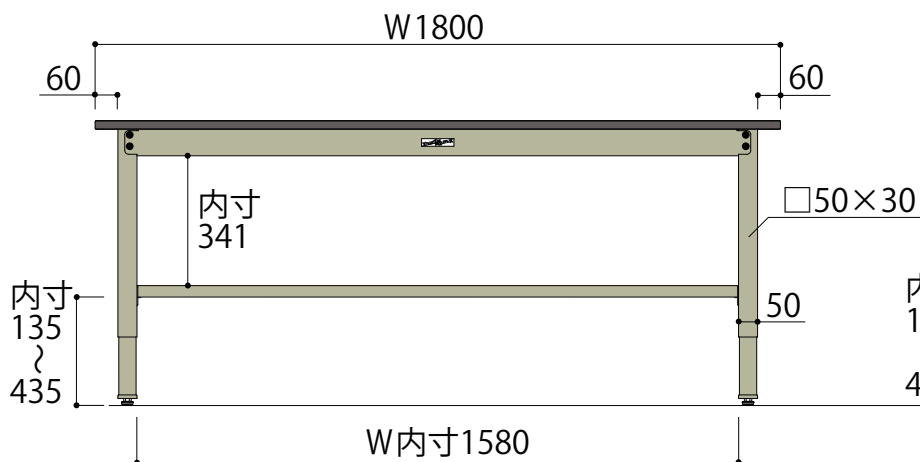
正面図
