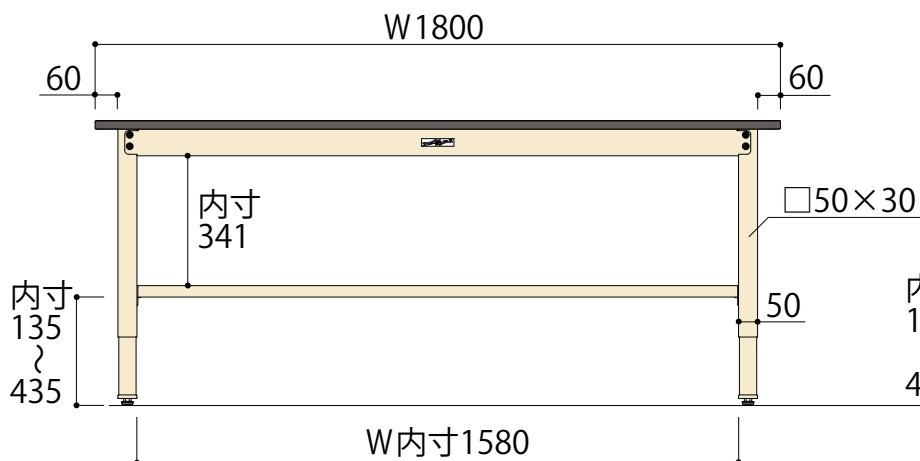
正面図
