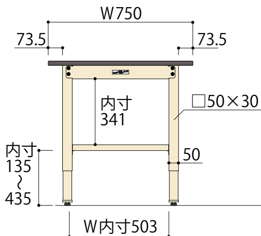
正面図
