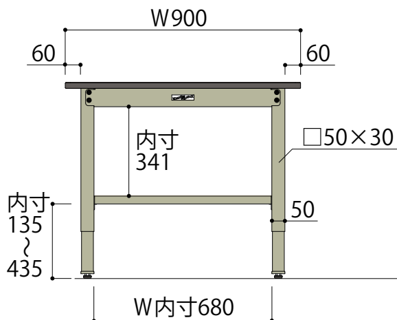
正面図
