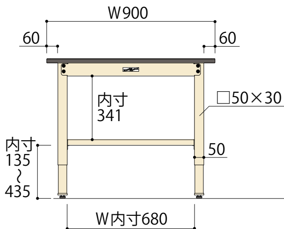
正面図
