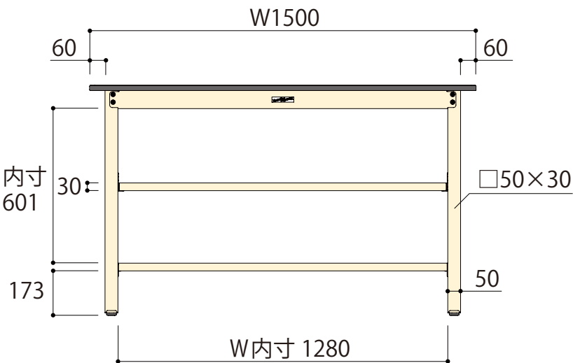
正面図
