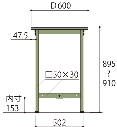
側面図
