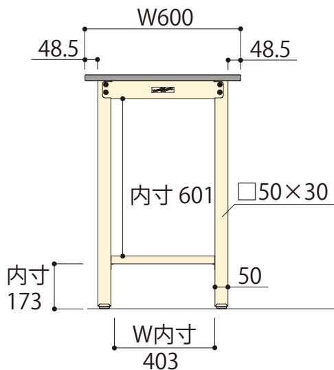
正面図
