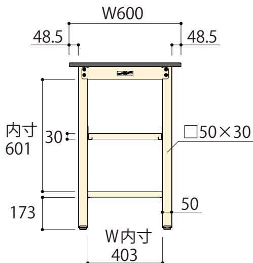
正面図
