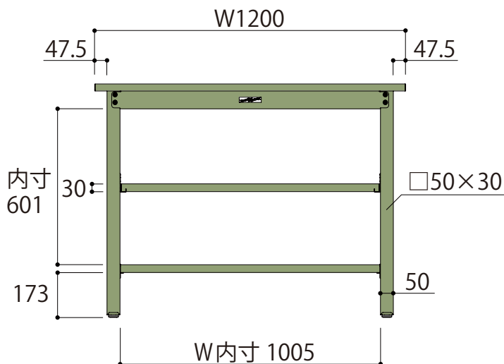
正面図
