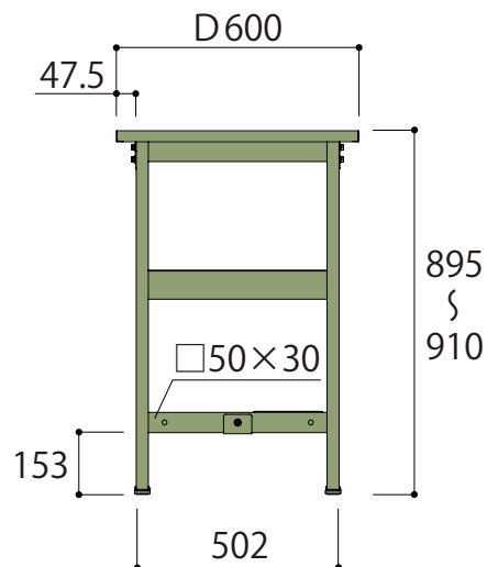
側面図
