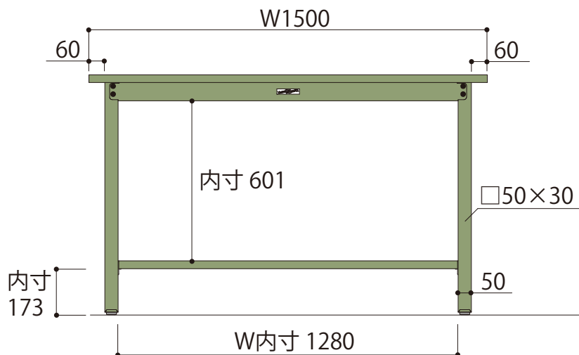
正面図
