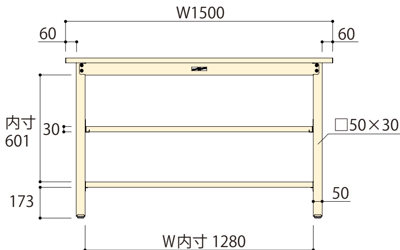
正面図
