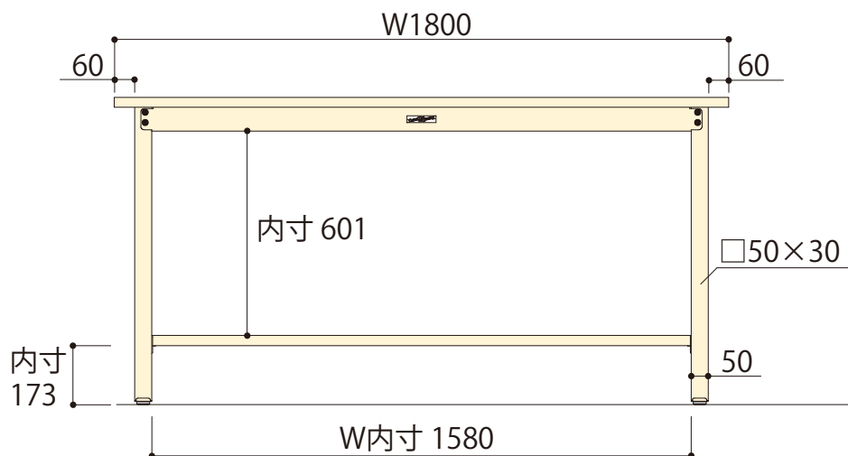
正面図
