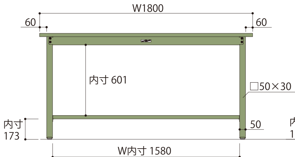
正面図
