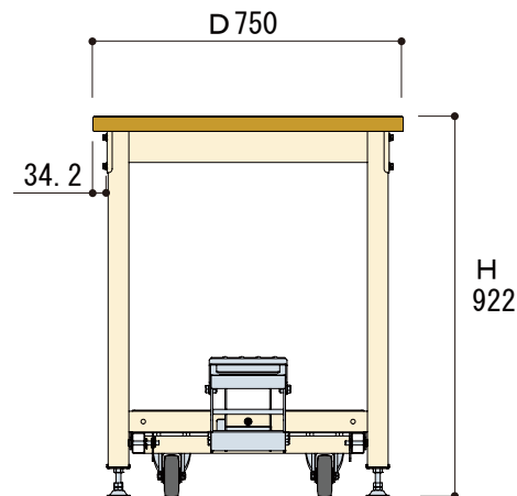
側面図
