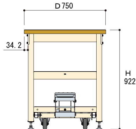
側面図
