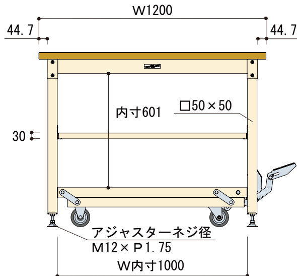
正面図
