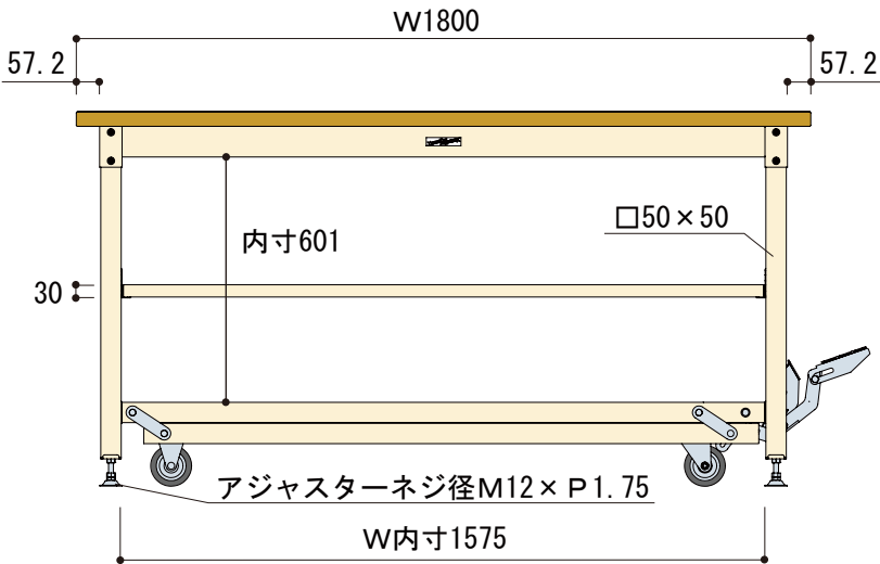
正面図
