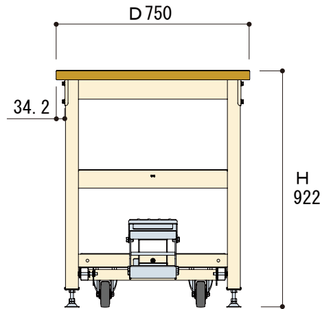
側面図
