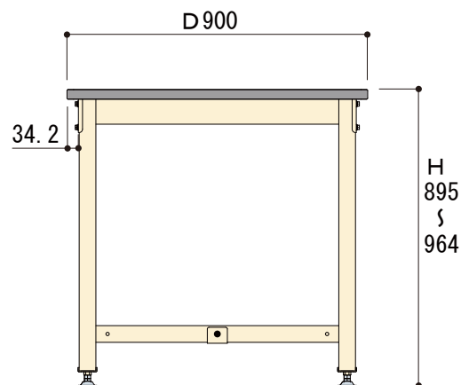
側面図
