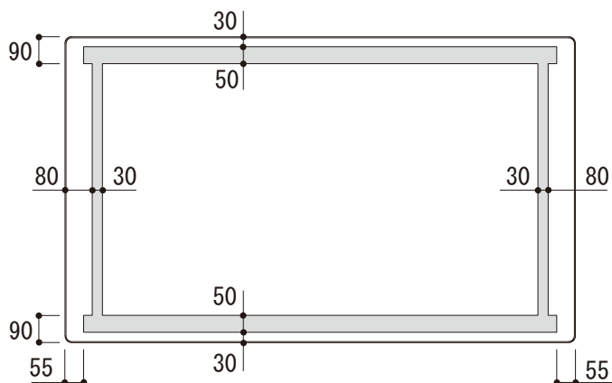
正面図
