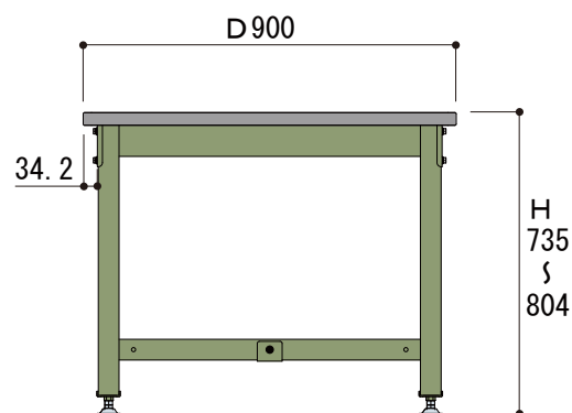
側面図
