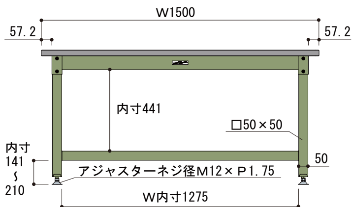
正面図
