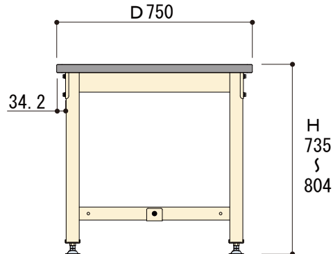
側面図
