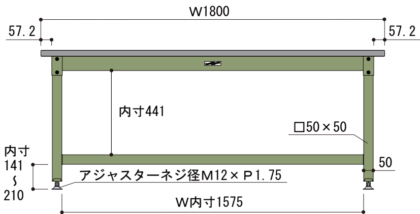
正面図
