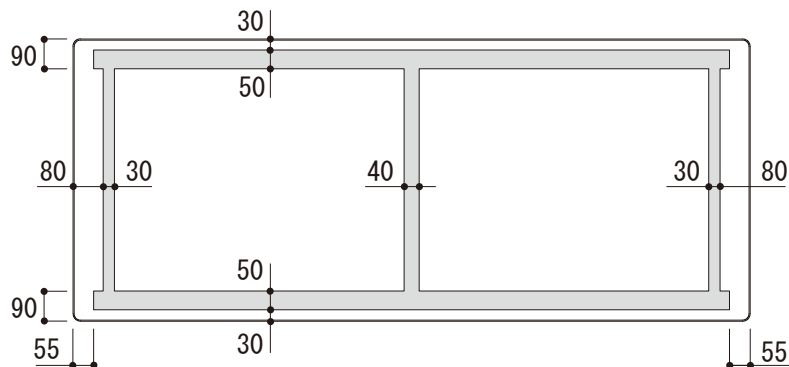
正面図
