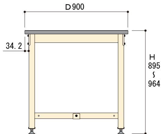
側面図
