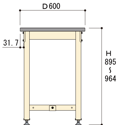
側面図
