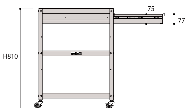
正面図
