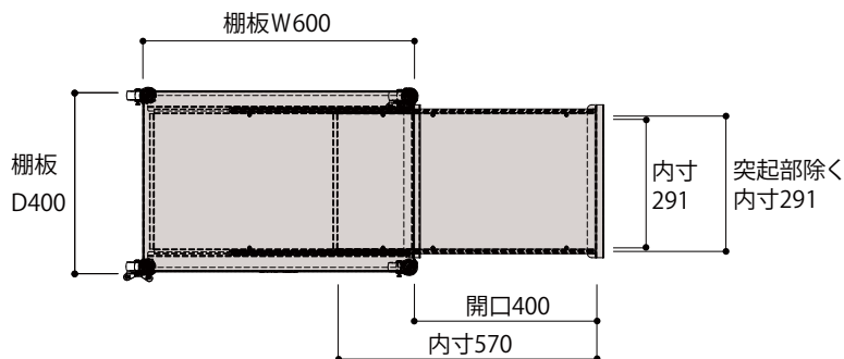
平面図
