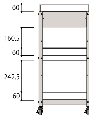
側面図
