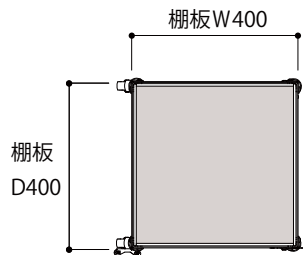
平面図
