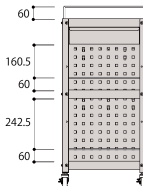
側面図
