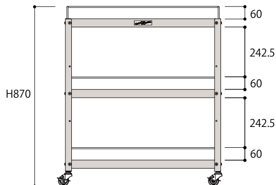
正面図
